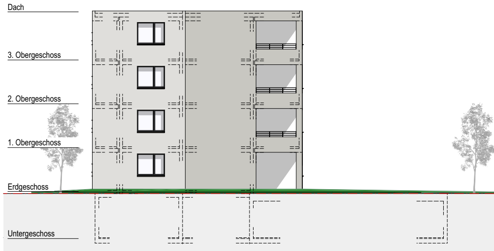
NORDFASSADE HAUS A
