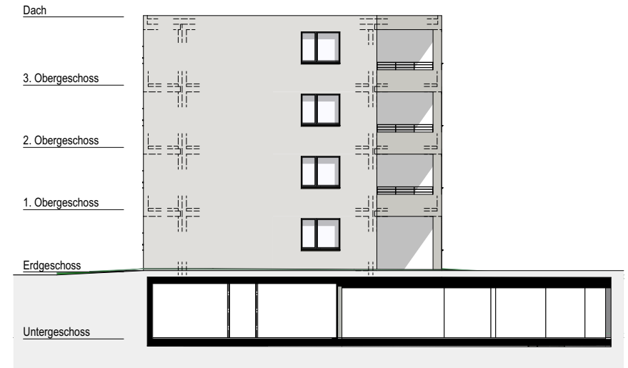
NORDFASSADE HAUS B
