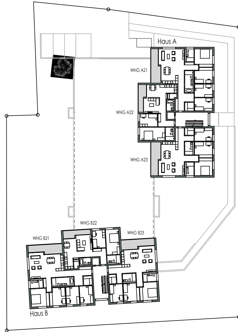
2. Obergeschoss
