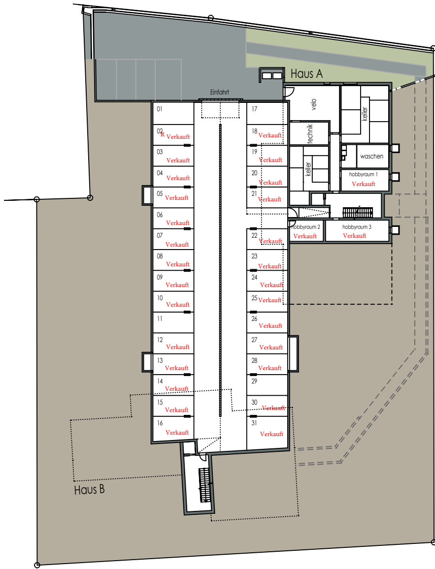
Untergeschoss
